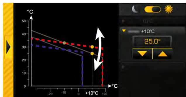
Fig. 5-51: Adapter la courbe de chauffage (en cas de températures extérieures supérieures à zéro).
