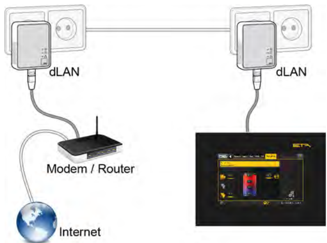
Fig. 5-31: Réseau dLAN
