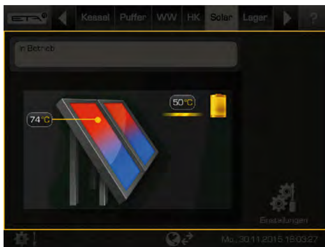
Fig. 5-59: Installation solaire avec échangeur de chaleur externe raccordé au ballon tampon
