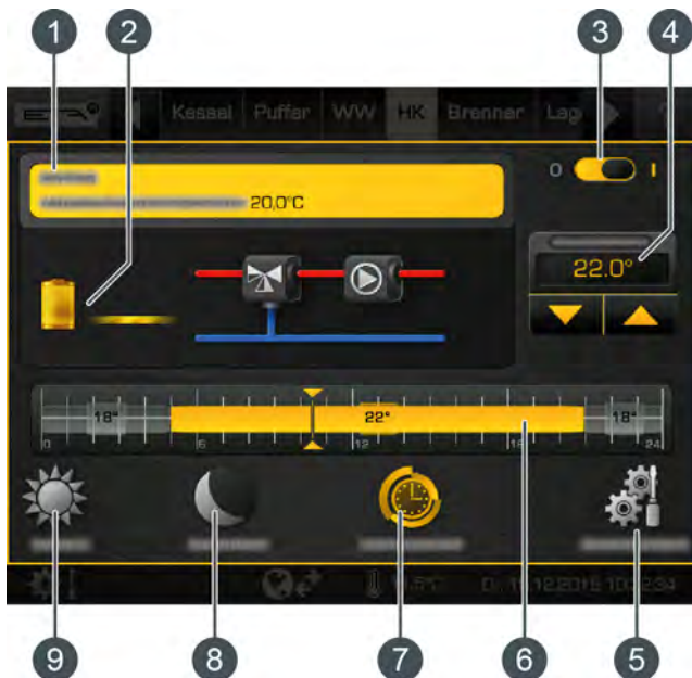
Fig. 5-43: Circuit de chauffage avec sonde d'ambiance
